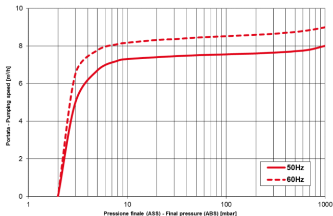
NOTA: Curve riferite alla pressione di aspirazione e temperatura 20°C (tolleranza ±10%)
